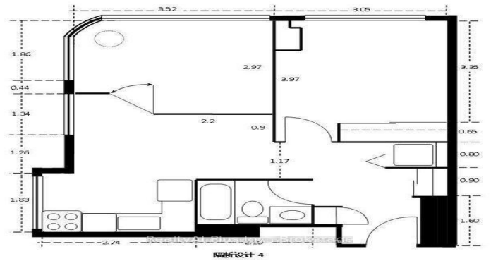
隔斷设计 4
